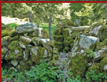
Un des ingénieux passages en Z ouvert dans l'un des murs latéraux d'un boviduc: forme et dimensions permettent le passage d'une personne, mais pas d'un bovin.
